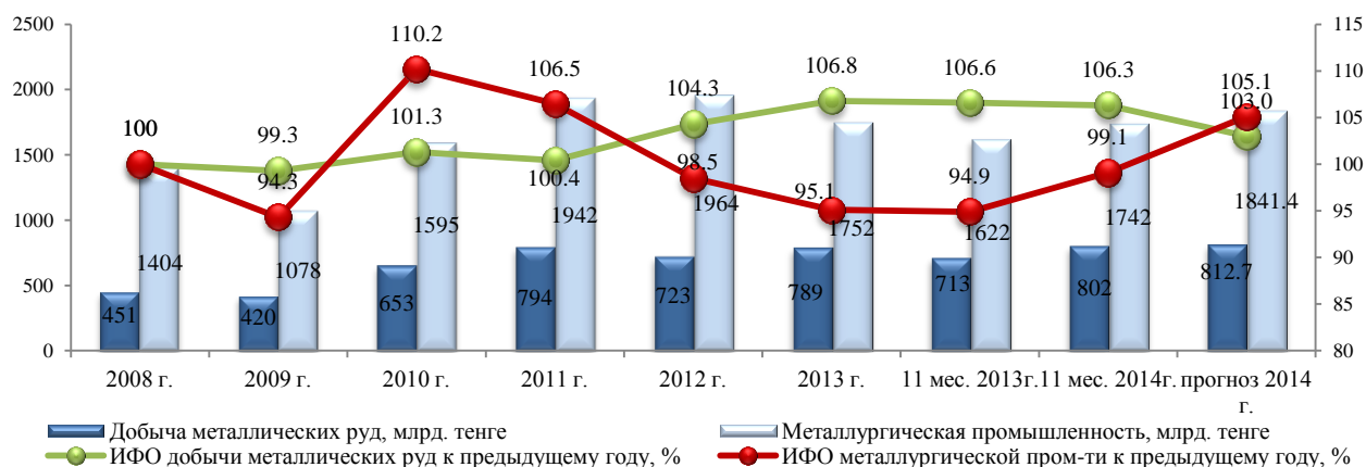
Рис. 1 Объёмы производства горно-металлургического комплекса, за 2008-2014 годы
